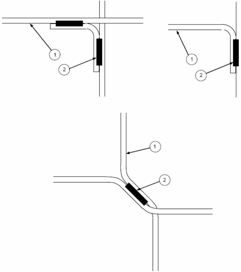
1 – арматурные стержни; 2 – сварное соединение длиной не менее 30 мм
