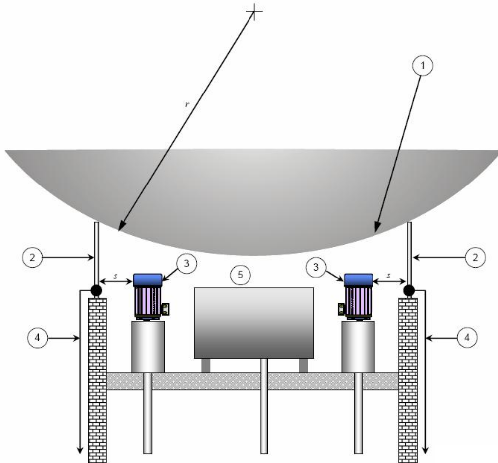
1 – катящаяся сфера; 2 – стержень молниеприемника; 3 – электрооборудование; 4 – токоотвод; 5 – металлический резервуар; r – радиус катящейся сферы, см. таблицу 2 настоящего предстандарта; s – безопасное расстояние согласно 6.3 настоящего предстандарта
