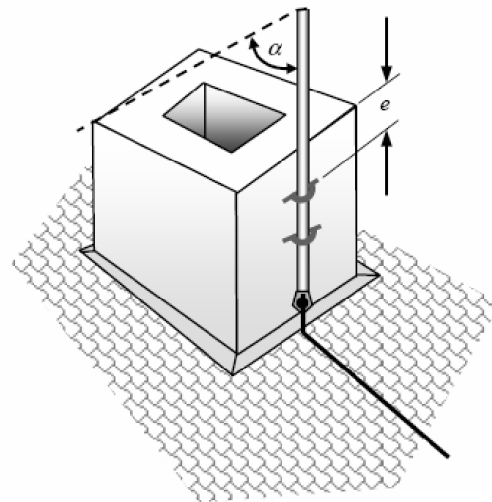
Рисунок Е.23б – Установка стержневого молниеприемника для защиты дымохода по методу защитного угла
