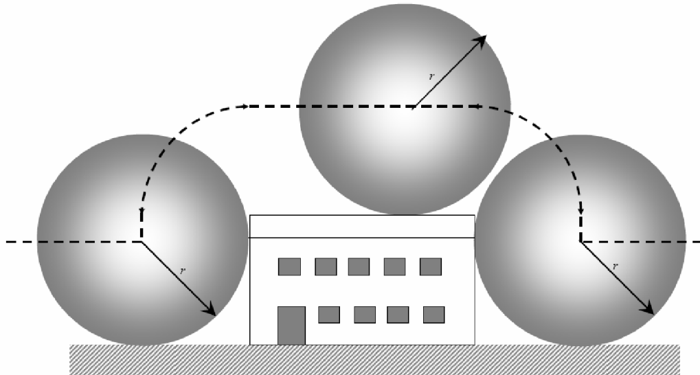
Рисунок Е.21а – Вид сбоку
