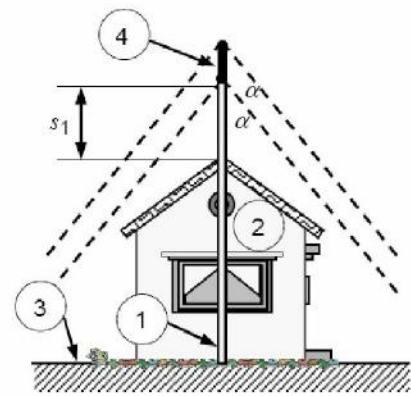
Рисунок Е.14б – Проекция на вертикальную плоскость, перпендикулярную плоскости, содержащей две мачты
