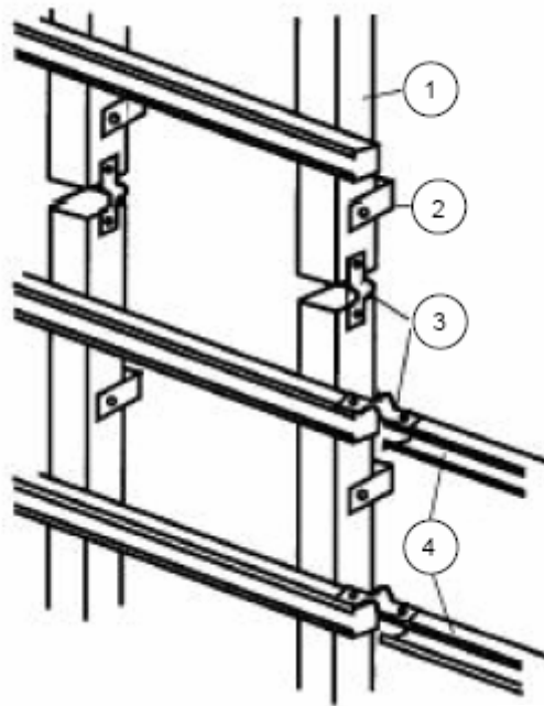
Рисунок Е.8b – Соединение опор фасада
