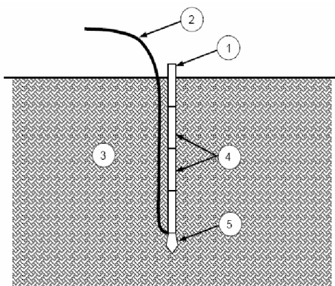
1 – короткий направляющий стержень; 2 – заземляющий проводник; 3 – земля; 4 – короткие направляющие стержни; 5 – направляющее стальное острие
