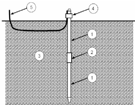
1 – увеличенный стержень заземления; 2 – стержневая муфта; 3 – земля; 4 – проводник для зажима стержня; 5 – проводник заземления
