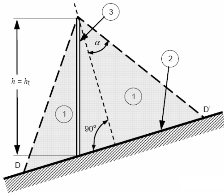
Рисунок Е.17б – Защищенное пространство стержня молниеприемника на наклонной поверхности при проектировании с использованием метода защитного угла
