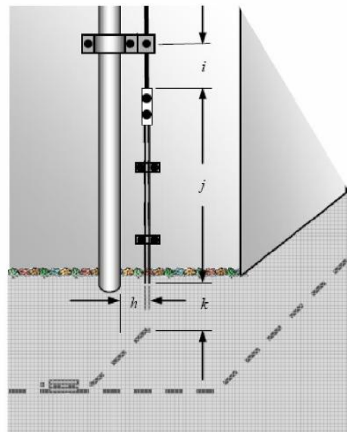
Рисунок Е.23д – Установка контрольного стыка в токоотводе и соединение с водосточной трубой
