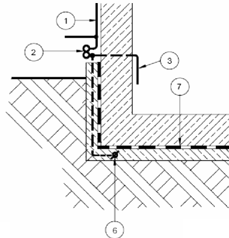
Рисунок Е.40b – Изолированный фундамент с проводником заземлителя, частично проходящим через землю
