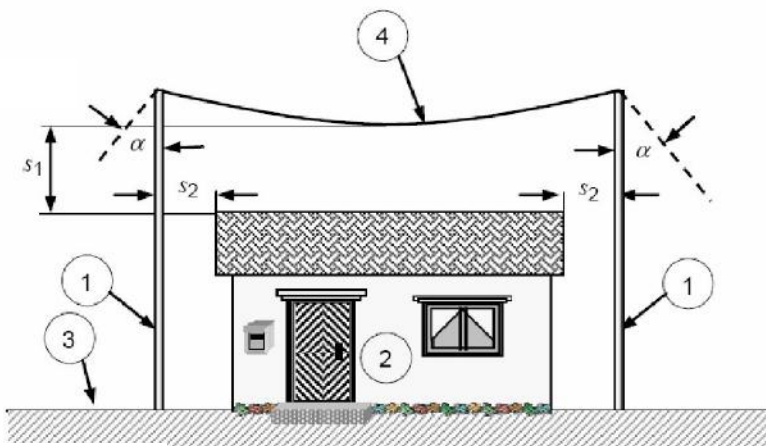
Рисунок Е.14а – Проекция на вертикальную плоскость, содержащую две мачты
