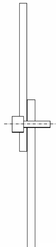
Рисунок Е.35b – Шунтирование гибкими самонарезающими винтами
